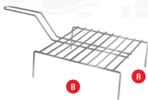
GRELHA COM PÉS N.º1: A265xB245mm N.º2: A300xB295mm N.º3: A385xB295mm
