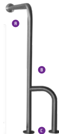
BARRA APOIO PAREDE SOLO 3 PONTOS MATERIAL: TUBO INOX 35x1.5 ACABAMENTO: ESCOVADO/BRANCO A750xB859xC200mm
