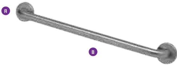
BARRA APOIO RECTA MATERIAL: TUBO INOX 35x1.5 ACABAMENTO: ESCOVADO/BRANCO A100xB300/400/500/600/800/1000mm
