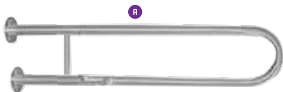
BARRA APOIO FIXA MATERIAL: TUBO INOX 35x1,5 ACABAMENTO: ESCOVADO/BRANCO A600/800mm
