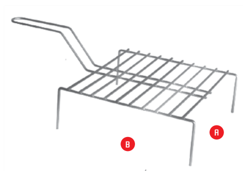
GRELHA c/PÉS N.º 1: A265x8245mm N.º 2: A300x8295mm N.º 3: A385x295mm
