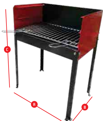
BARBECUE STYLE VERMELHO A500x8300xC670mm
