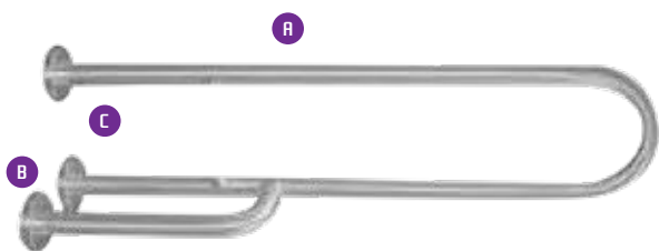
BARRA APOIO FIXA 3 PONTOS MATERIAL: TUBO INOX 35x1,5 ACABAMENTO: ESCOVADO/BRANCO A600/800x8175xC210mm
